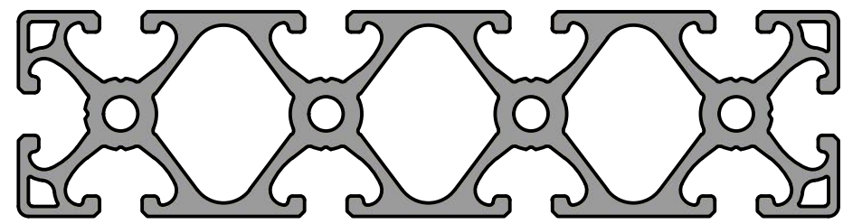
Sichtfläche/ visible surface SCALE= ( 1 : 1 )
